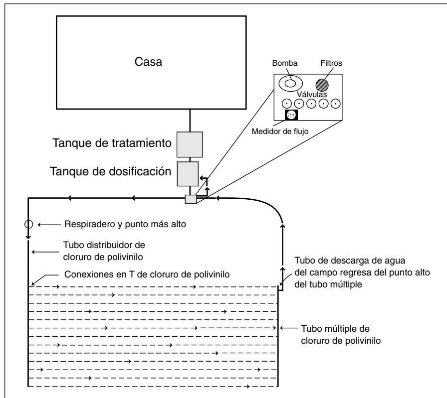
Figura 3: un sistema de distribución por goteo para el tratamiento y su dispersión.
